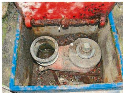
Bouche Incendie de 80 mm à raccord Keyser
