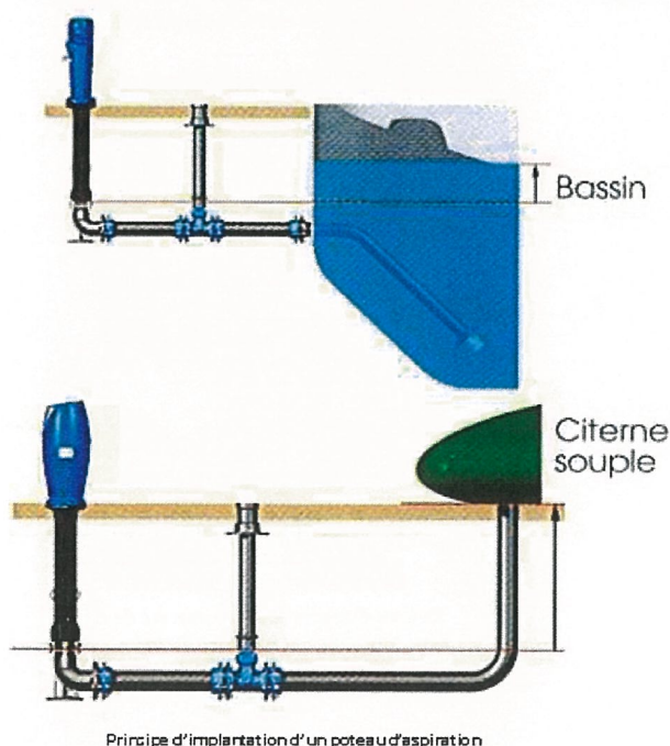
Principe d'implantation d'un poteau d'aspiration
