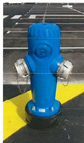
Poteau d'aspiration à réseau sec de 150 mm, muni de deux sorties de 100 mm et d'un Aircap. Pas de carré ni de volant de manœuvre
